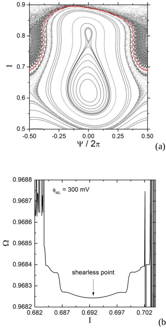
Figura 6.7: Mapa de Poincaré (a) ao considerar a amplitude do potencial flutuante \phi_{ML} = 300 \text{ mV} , perfil de velocidade paralela não-uniforme e perfil não-monotônico do fator de segurança. A curva sem cisalhamento está destacada na cor vermelha e foi determinada pelo mínimo do perfil do número de rotação apresentado em (b).
