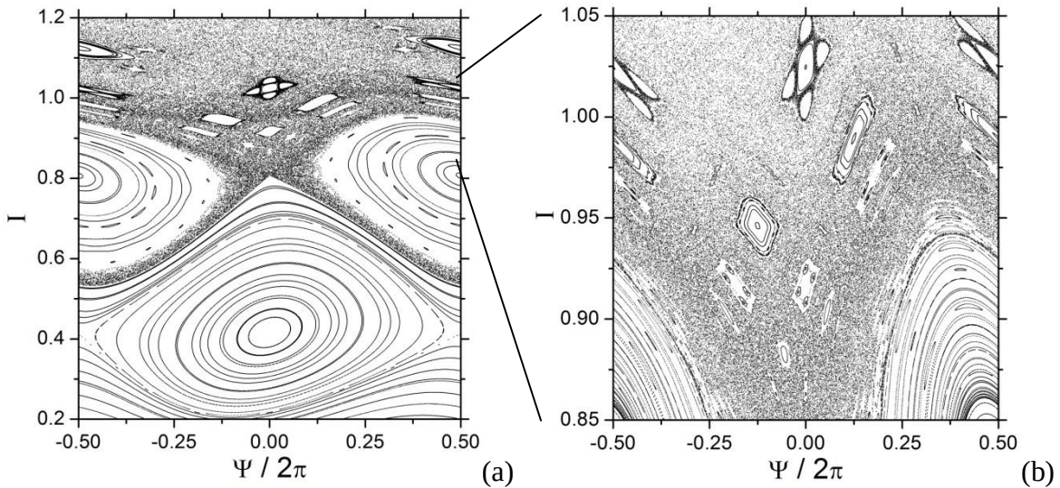
Figura 5.4: Mapa simplético (a) para um potencial flutuante \phi_{ML} = 0.65 \text{ V} e (b) o mesmo mapa ampliado na borda do plasma.
