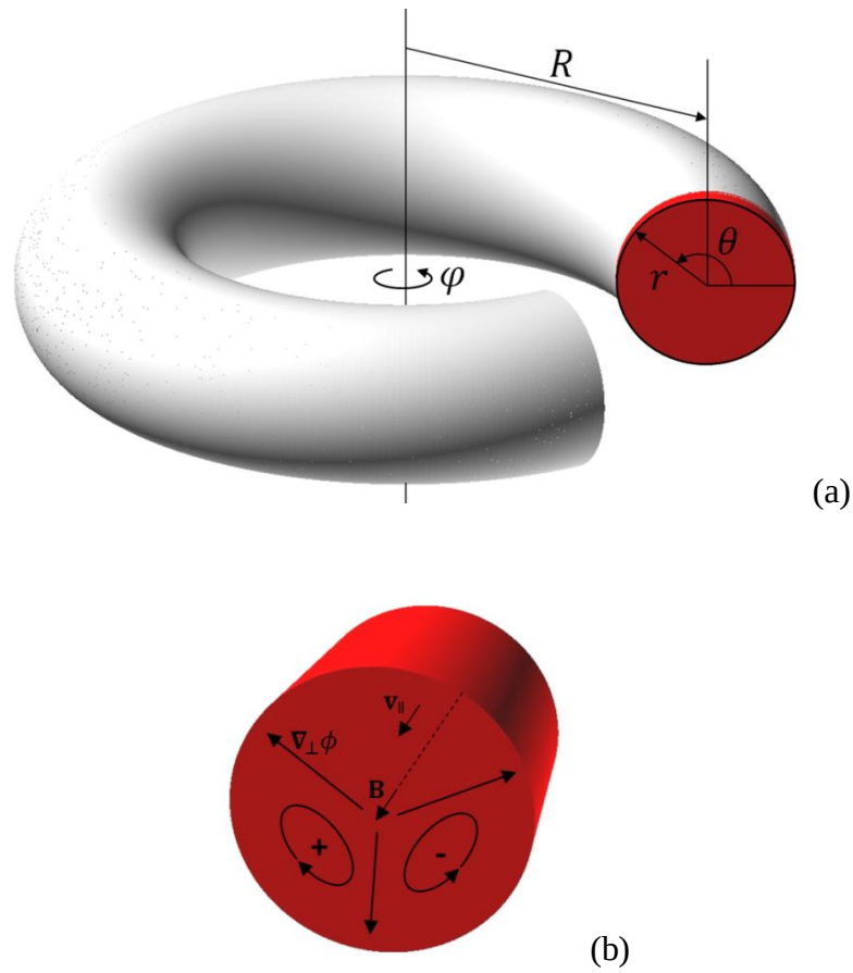
Figura 2.1: Seção transversal de um toróide (a) com as coordenadas locais polares no segmento em vermelho e a representação da trajetória das partículas do plasma (b) com as grandezas vetoriais do campo magnético, da componente do potencial eletrostático perpendicular ao campo magnético e da velocidade paralela.
