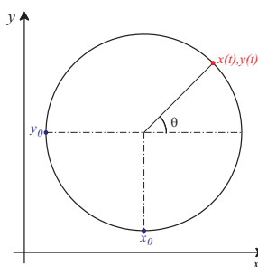
Figura 1: Ilustração da determinação de uma fase geométrica para o movimento sobre um ciclo limite atrativo descrito no plano de fase x, y , sendo x_0, y_0 , os pontos considerados no interior do plano de fase.
