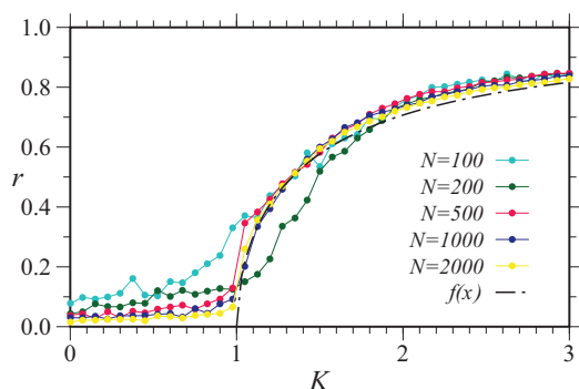
Figura 5: Módulo do parâmetro de ordem em função da intensidade de acoplamento em um sistema de N = 100, 200, 500, 1000 e 2000 osciladores de fase acoplados segundo o modelo de Kuramoto. A linha tracejada preta representa a previsão teórica (ver material suplementar) no limite de N grande.
