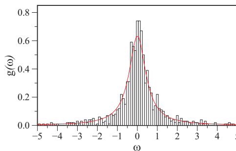
Figura 3: Histograma para as frequências naturais de N = 1000 osciladores de fase. A curva vermelha representa uma distribuição Lorentziana (26) com \gamma = 0,5 .
