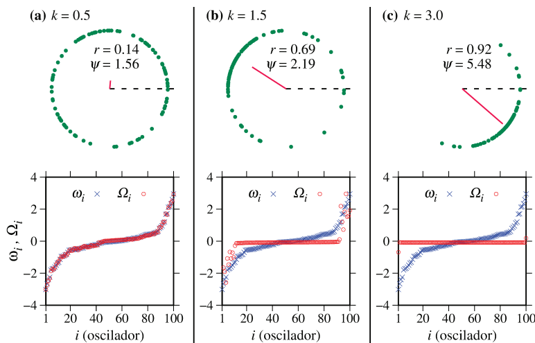
Figura 4: Fases (cor verde, acima) e frequências perturbadas (cor vermelha, abaixo) e não-perturbadas (cor azul, abaixo) para o modelo de Kuramoto com N = 100 osciladores nos casos (a) K = 0,5 ; (b) 1,5; (c) 3,0. Nos painéis acima indicamos os parâmetros de ordem correspondentes aos três casos.
