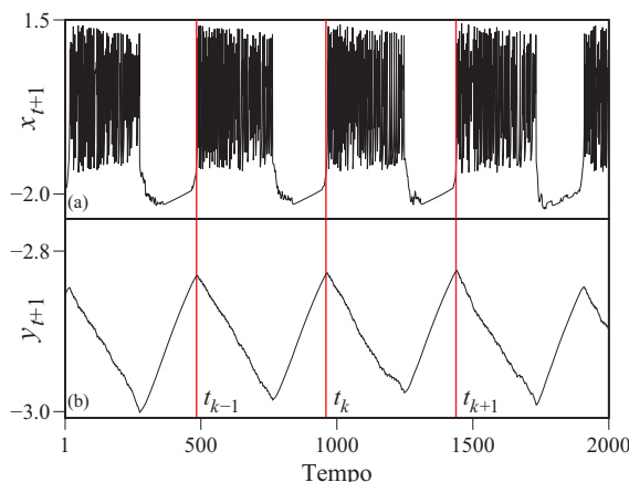
Figura 2: Evolução temporal da (a) variável rápida (relacionada ao potencial de membrana) e (b) variável lenta para um neurônio descrito pelo modelo de Rulkov (3)–(4).
