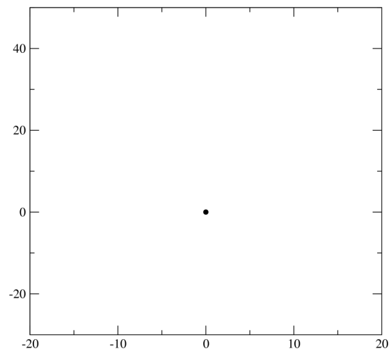
Figura 1 – Para r = 0 , a origem é ponto fixo estável
