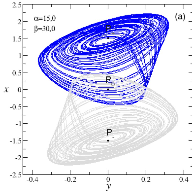
(a) Atratores coexistentes do tipo Rössler (b) Bacia de atração dos atratores em x = 0 .
