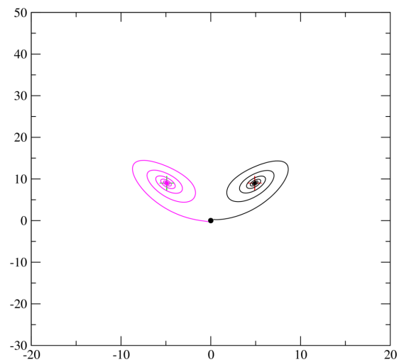
Figura 2 – Para r = 10 , a origem é ponto fixo instável e surgem dois outros pontos fixos estáveis C_+ e C_-
