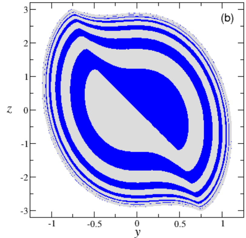
(a) Atratores coexistentes do tipo Rössler (b) Bacia de atração dos atratores em x = 0 .
