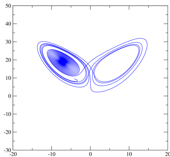
Figura 3 – Para r = 20 , existem órbitas caóticas não atratoras (transientes)
