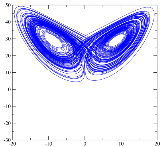
Figura 5 – Para r = 30 , só existe o atrator caótico
