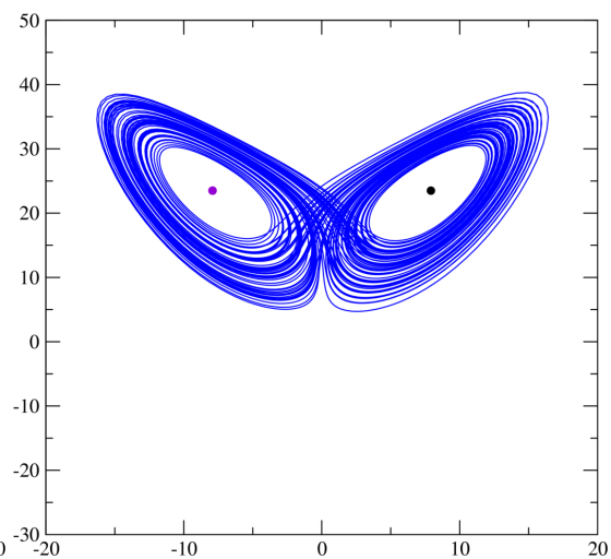
Figura 4 – Para r = 24.5 , coexistência do atrator caótico com os pontos fixos estáveis C_+ e C_-
